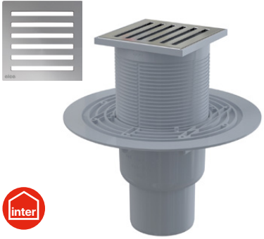
APV203 Padlóösszefolyó 105×105/50/75 mm függőleges, rozsdamentes rács, vizes búzzár
