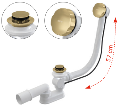
A55K-G-P Automata kádszifon készlet, GOLD-fényes
