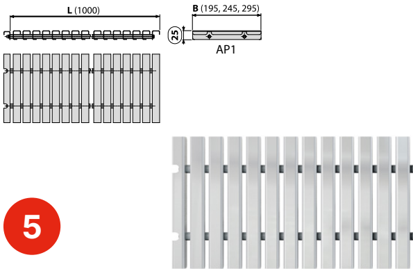
AP1 Medence rács csúszásgátló nélkül
