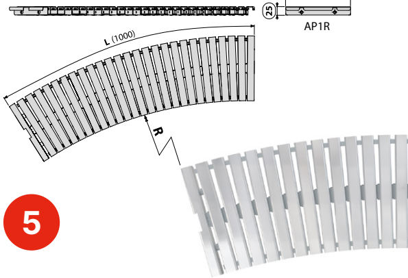
AP1R Íves medence rács csúszásgátló nélkül
