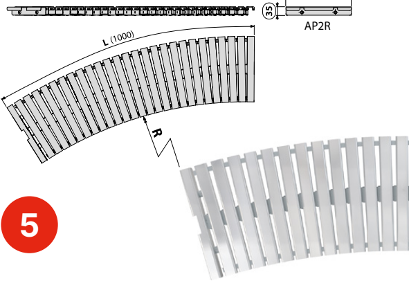
AP2R Íves medence rács csúszásgátló nélkül
