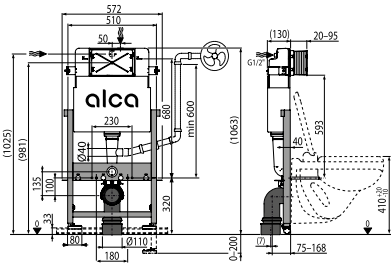
AS101 Sádromodul Falsík alatti szerelési rendszer száraz szereléshez (gipszkarton)
