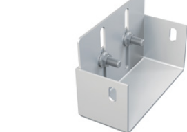
ADZ-P011 Drén folyóka véglezáró elem 75 mm, rozsdamentes acél
