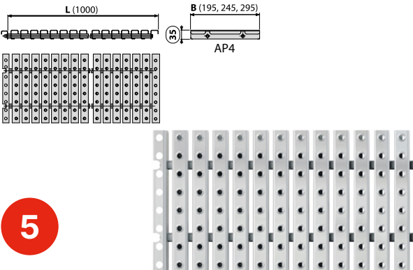
AP4 Medence rács csúszásgátlóval
