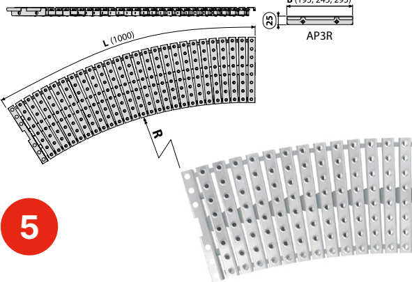
AP3R Íves medence rács csúszásgátlóval
