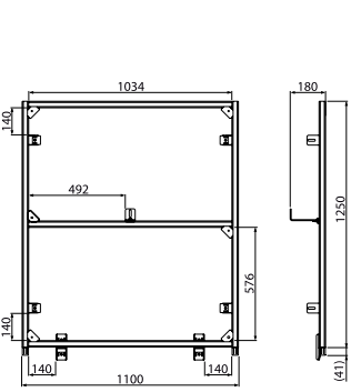
AS101-SET02, AS101-SET02-PR * Fal rendszer
