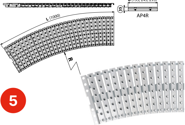
AP4R Íves medence rács csúszásgátlóval
