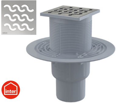
APV202 Padlóösszefolyó 105×105/50/75 mm függőleges, rozsdamentes rács, vizes búzzár
