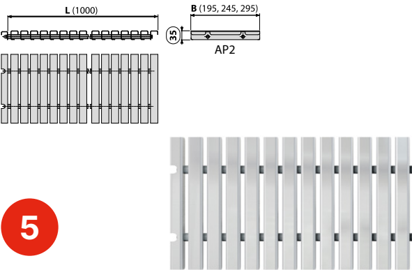
AP2 Medence rács csúszásgátló nélkül
