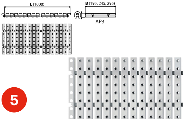
AP3 Medence rács csúszásgátlóval
