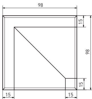
piesă colț de duș cu pantă / shower piece - corner | GTRON... | 98×98×6 mm
