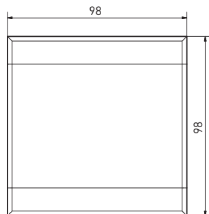
piesă de duș cu pantă / shower piece - continuous | GTPON... | 98×98×6 mm
