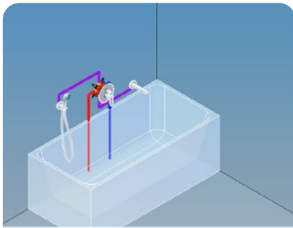
Süllyesztett kétutas csaptelep, fali csatlakozós kézzzuhany tartó, kád kifolyócső
