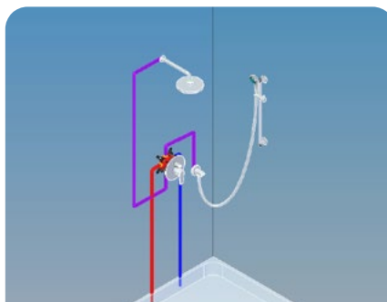
Süllyesztett kétutas csaptelep, zuhanyezett zuhanyrúddal, fali csatlakozós kézzzuhany tartó, zuhanykar, Evo zuhanyfej
